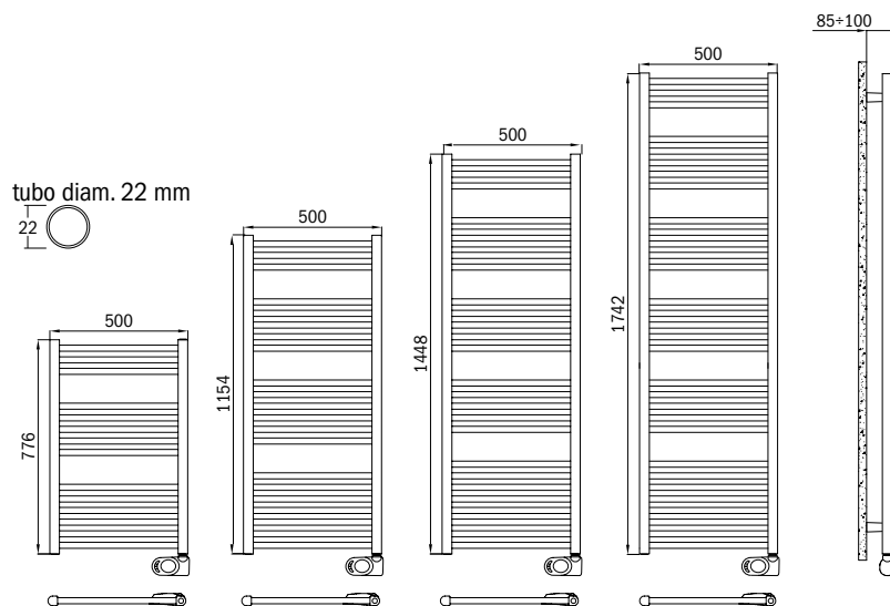
quote in mm - collettori semiovali 40x30
